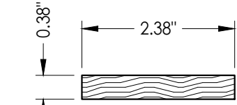
16 JAMB EXTERIOR SASH STOP
